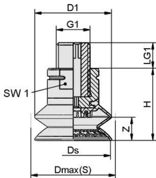
设计参数 SAXB 20 ED-85 M16-AG
