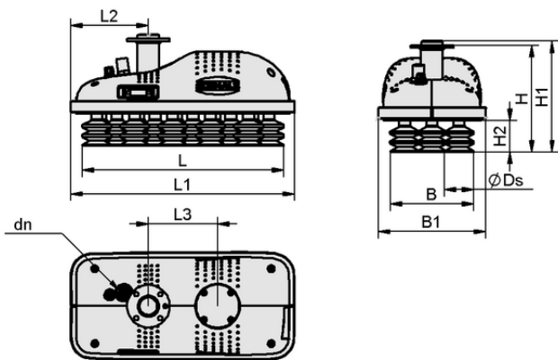
设计参数 ROB-SET FXCB FANUC SPB2
