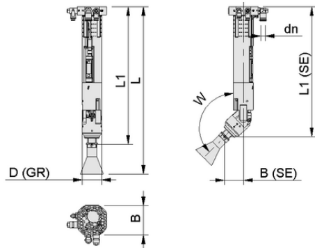
设计参数 SBPG X PSE 312 50 SVE
