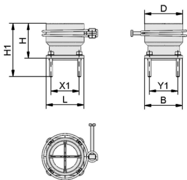
设计参数 SCHL-AN 32.5-47x47x48 PSSG
