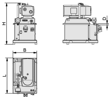
设计参数 VH-TR Plus 25 30
