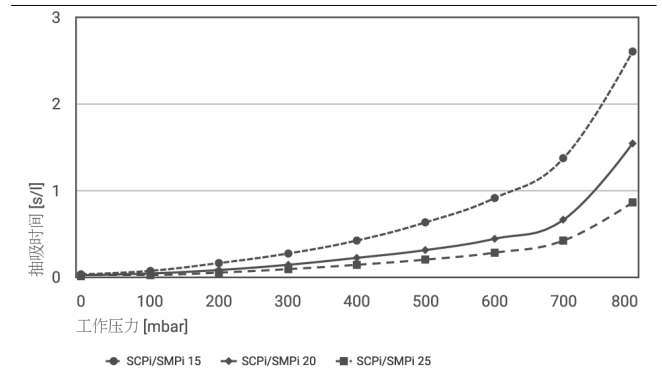
不同真空范围的抽吸时间 [s/l]
