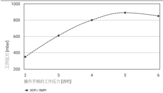
在不同工作压力下实现，达到的真空度
