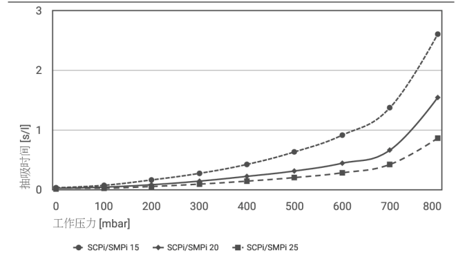
不同真空范围的抽吸时间 [s/l]
