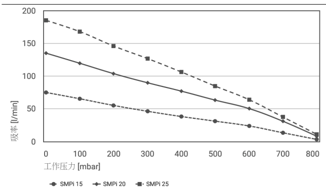
不同抽真空度下的吸率[升/分钟]
