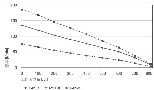
不同抽真空度下的吸率[升/分钟]
