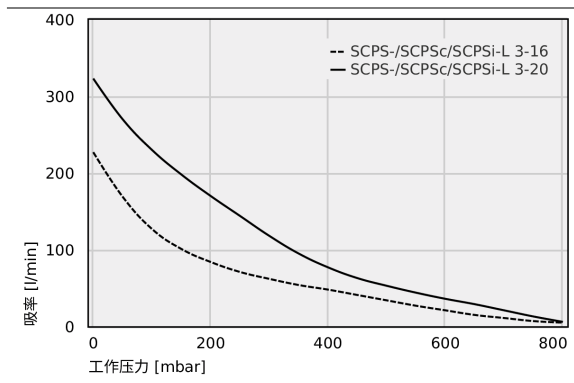
不同抽真空度下的吸率[升/分钟]
