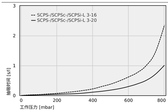
不同真空范围的抽吸时间 [s/l]
