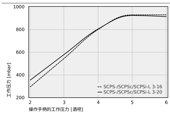
在不同工作压力下实现，达成的真空度
