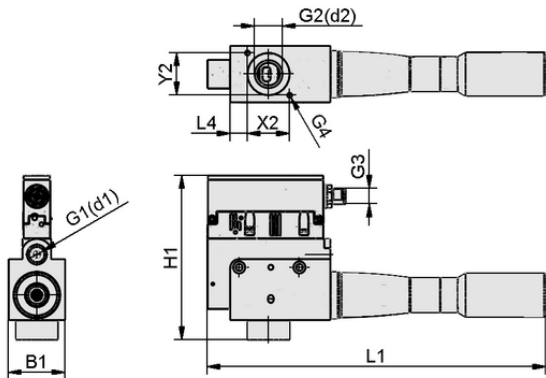
设计数据 SCPS-L HV 3-20 NC M12-5 PNP
