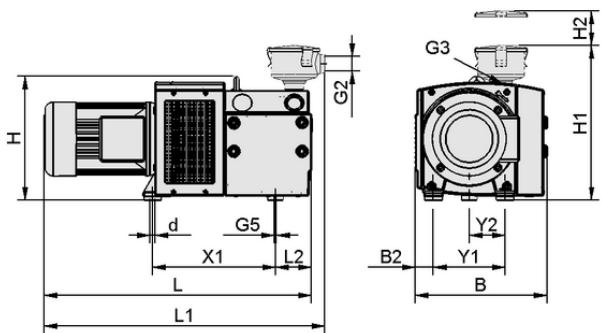
设计参数 EVE-TR 60 AC3 IE3-TYP2
