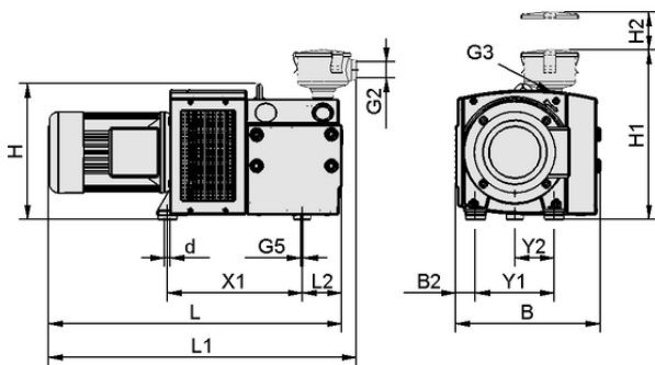
设计参数 EVE-TR 80 AC3 IE3-TYP2
