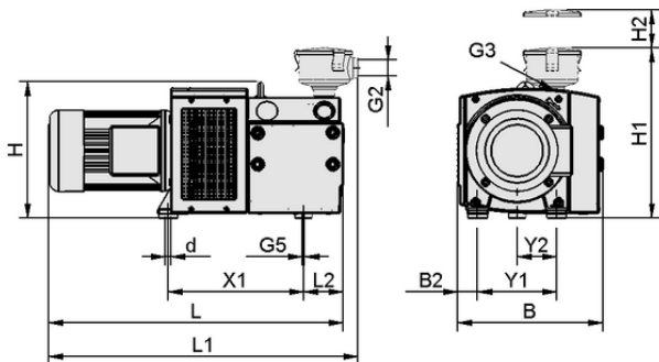
设计参数 EVE-TR-X 80 AC3 IE3-TYP1 VBV
