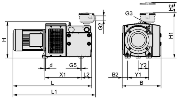
设计参数 EVE-TR-X 100 AC3 IE3-TYP1 VBV
