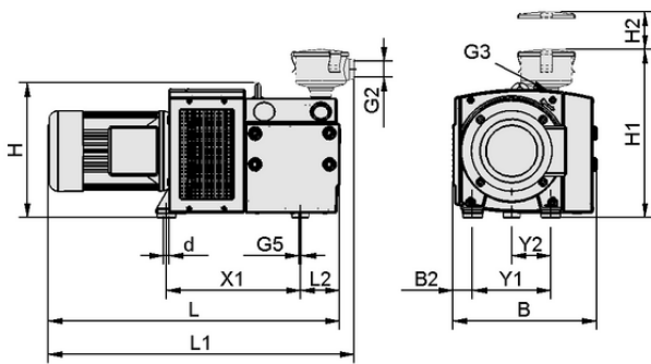
设计参数 EVE-TR-X 80 AC3 IE3-TYP2 F-VB
