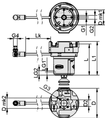
Design data ROB-SET ECBPMi MIT
