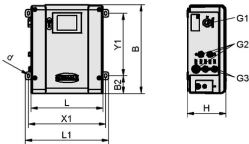
设计参数 GCPI 50 5xM12-5 24V-DC
