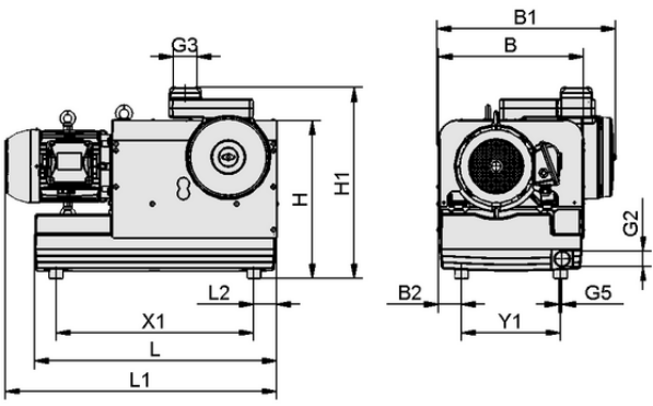
设计参数 EVE-KL 150 AC3 FU
