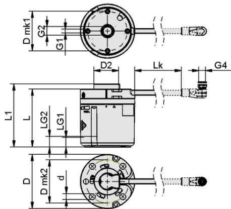
设计参数 ROB-SET ECBPMi JAKA
