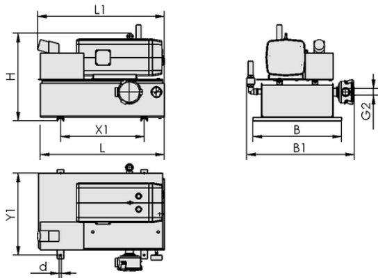
设计参数 VZ-OG 63 AC3 100 GMS
