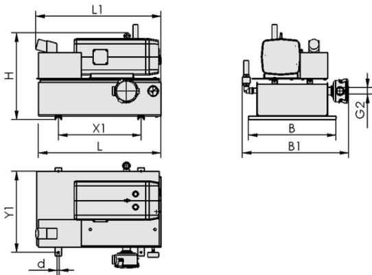
设计参数 VZ-OG 63 AC3 100
