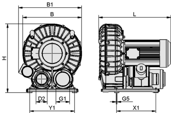
设计参数 SB 510 390 11 IE3-TYP3
