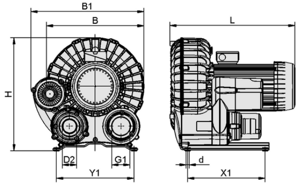
设计参数 SB 235 400 3.6 IE3-TYP4
