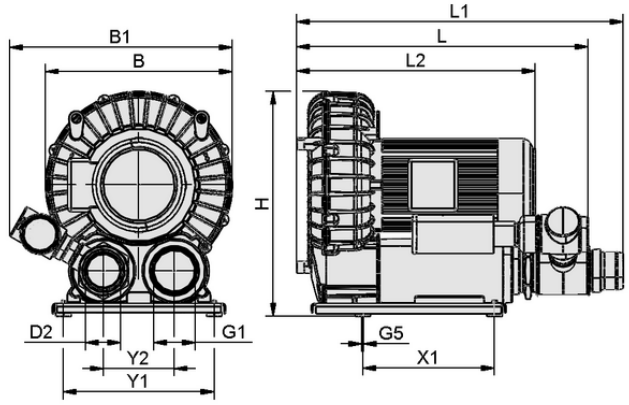
设计参数 SB 765 280 7.5 IE3-TYP1
