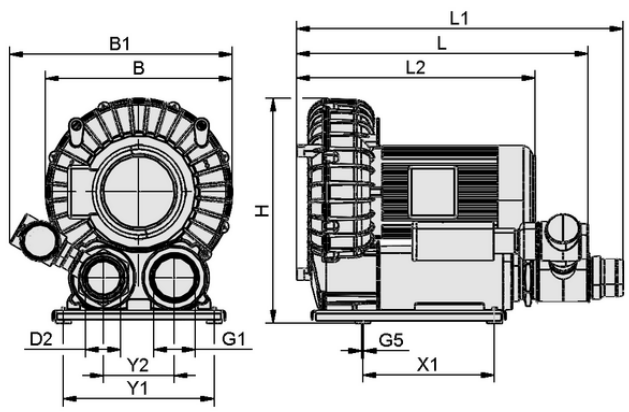
设计参数 SB 1050 290 11 IE3-TYP1
