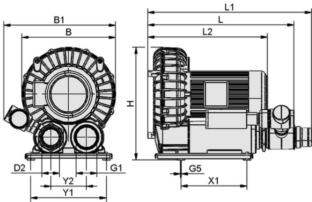
设计参数 SB 375 390 5.5 IE3-TYP1
