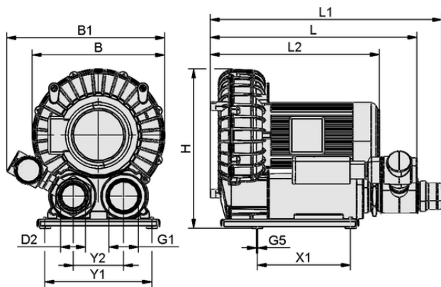
设计参数 SB 435 340 6.6 IE3-TYP2
