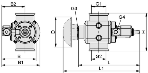
设计参数 EMVP 50 24V-DC 3/2 NC
