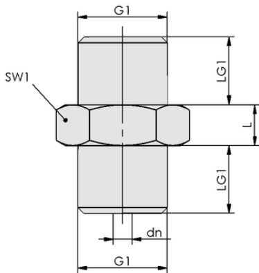
设计参数 SW 50 G1/8-AG
