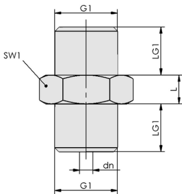
设计参数 SW 120 G1/8-AG
