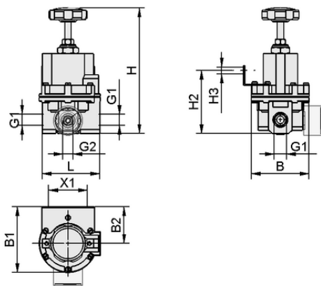
设计参数 VR G3/8-IG HW
