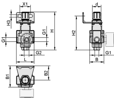
设计参数 VR G1/4-IG HW
