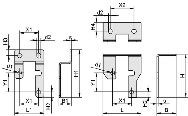
设计数据 BEF-WIN 13x50x31 1.6 VS
