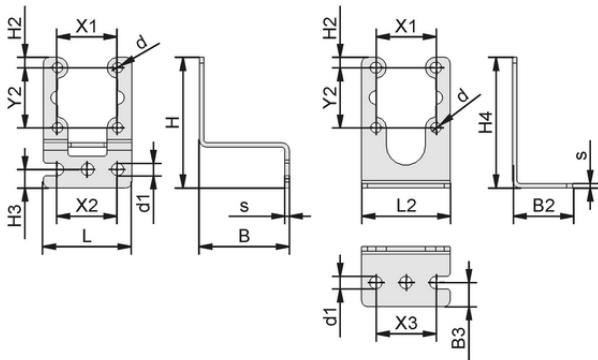
设计参数 BEF-WIN 30x43.5x29.5 1.5
