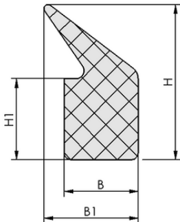
设计参数 DI-PROF 11x23 MOS CR-20 DL
