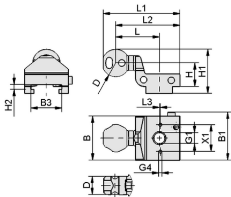
设计参数 HT-SG A2 E 46 RA
