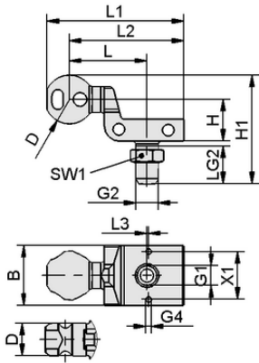
设计参数 HT-SG A3 E 35 NPT1/4-AG
