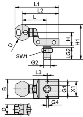
设计参数 HT-SG A3 E 35 NPT3/8-AG
