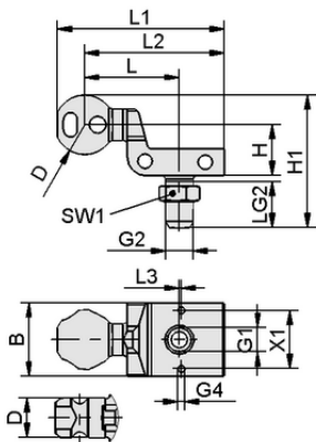
Design data HT-SG A5 E 35 G3/8-AG
