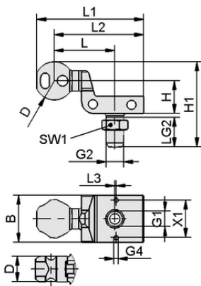
设计参数 HT-SG A2 E 35 G3/8-AG
