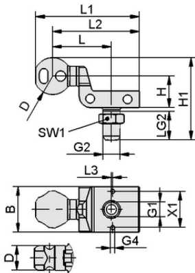
Design data HT-SG A2 E 35 G3/8-AG
