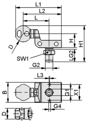
设计参数 HT-SG A2 E 35 NPT3/8-AG
