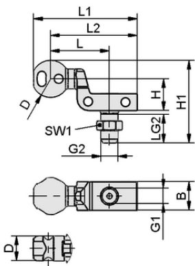
设计参数 HT-SG A2 22 NPT1/4-AG
