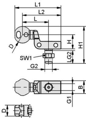
设计参数 HT-SG A5 22 NPT3/8-AG
