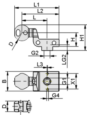
Design data HT-SG A5 E 35 M10-IG
