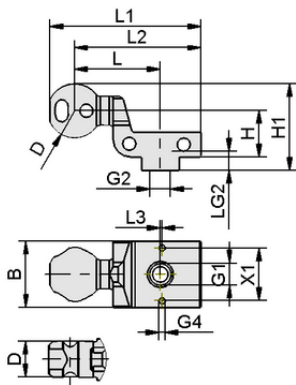
设计参数 HT-SG A2 E 35 M14x1.5-IG
