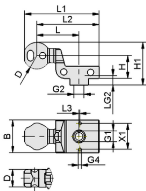
Design data HT-SG A2 E 35 M16x1.5-IG
