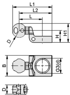
设计参数 HT-FST A2 35 M20x1.5
