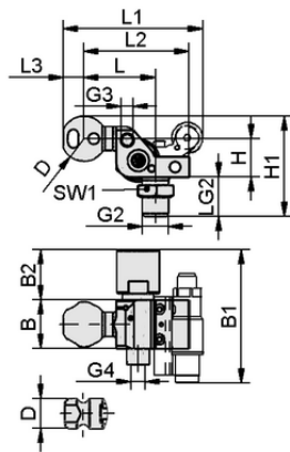
设计参数 HT-SG A3 I 10 31 NPT3/8-AG AB
