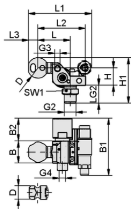
设计参数 HT-SG A5 I 10 31 G3/8-AG AB VS
