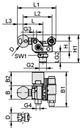
设计参数 HT-SG A2 I 10 31 NPT3/8-AG AB VS
